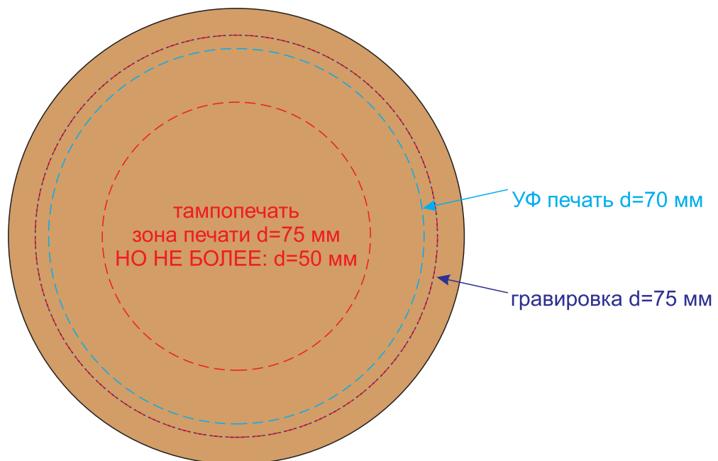
крышка
